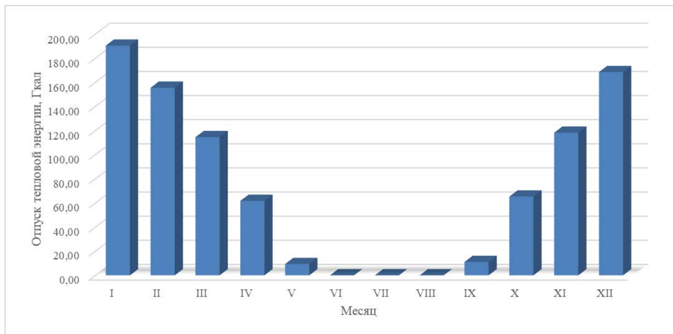
Рисунок 1.2 – Оптимальный температурный график отпуски тепловой энергии по котельной с. Назино
